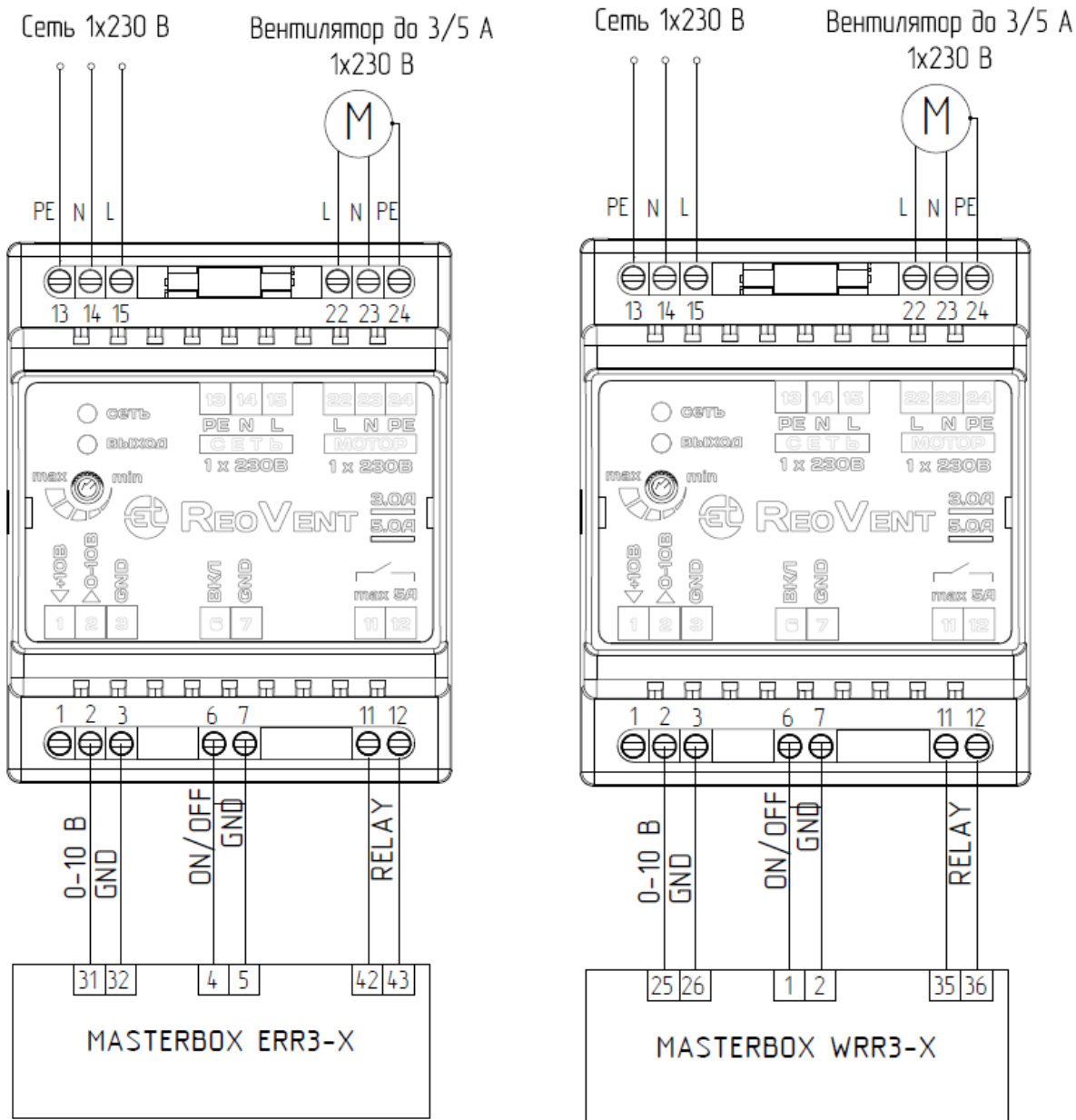
Рис. 2 Подключение регулятора Reovent к шкафам автоматики Masterbox RR3
