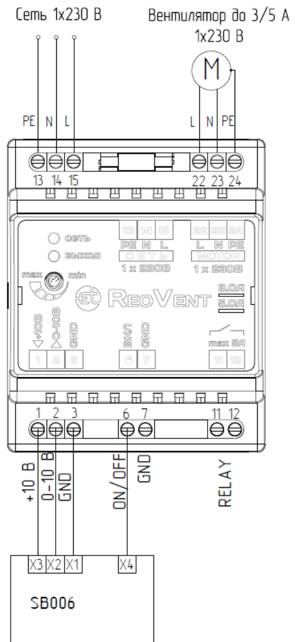
Рис. 4 Подключение регулятора Reovent к внешнему задатчику SB006
