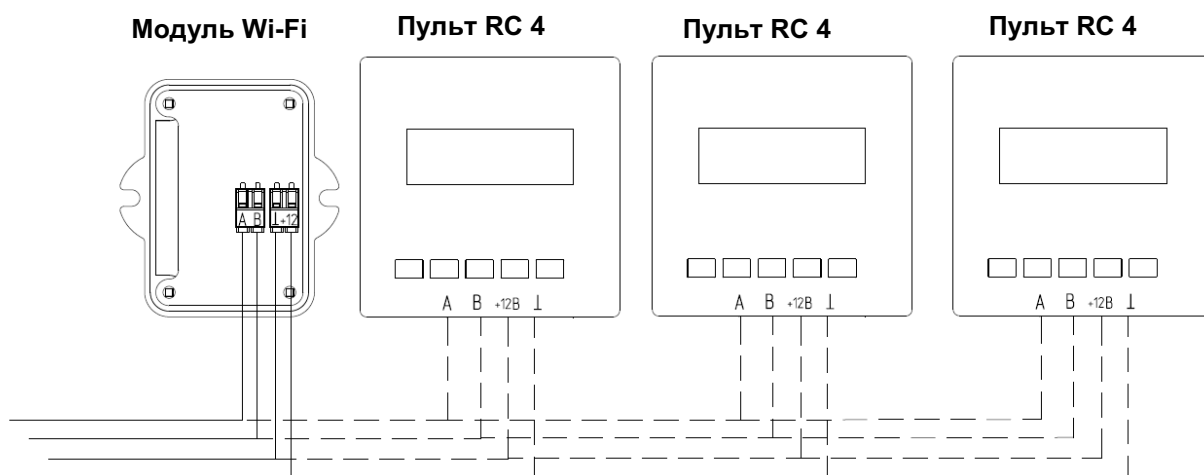
Рис. 7 Подключение одного модуля Wi-Fi и трех пультов RC 4
